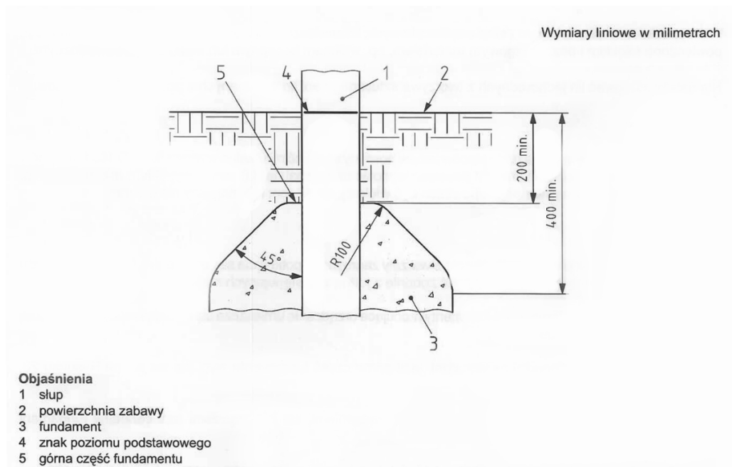
Rys. Fundamentowanie urządzeń placu zabaw wg PN-EN 1176-1:2009
